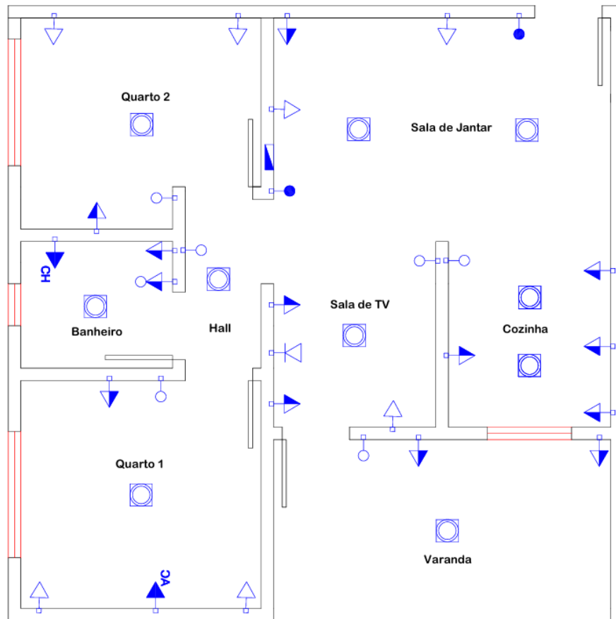
Figura 5 - Representação dos pontos de tomada e iluminação
